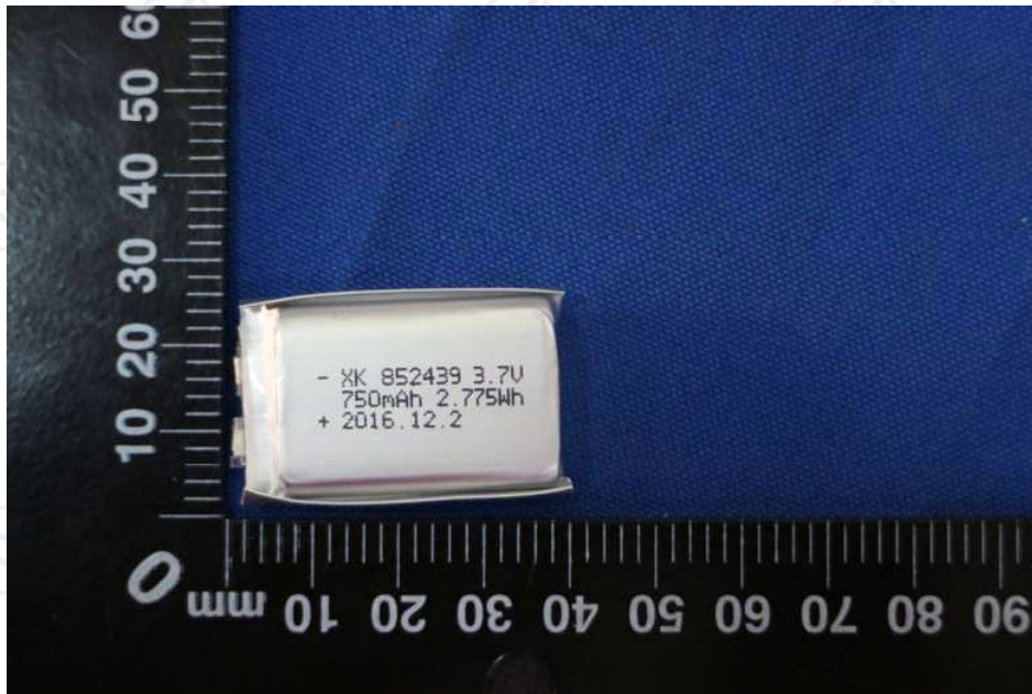
Photo 3 Internal Cell 内部电芯
